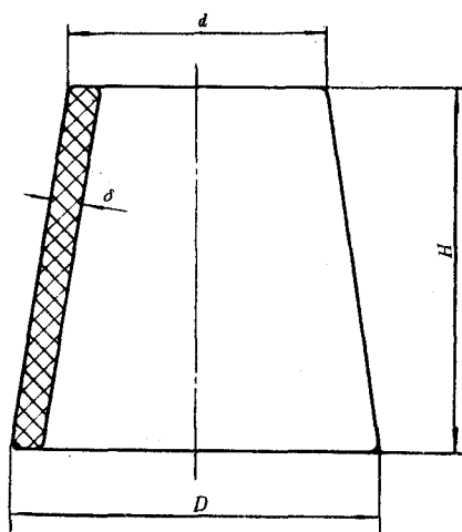
图 2 圆锥形瓷套
