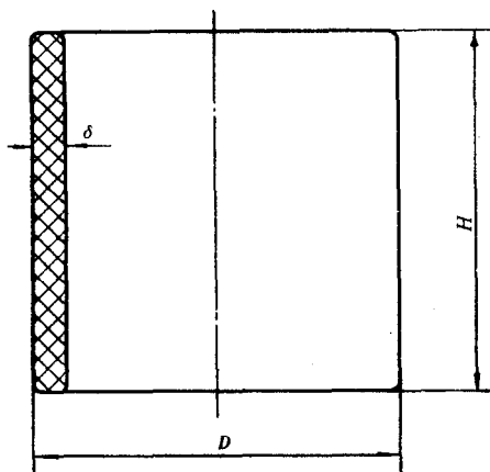
图 1 圆柱形瓷套
